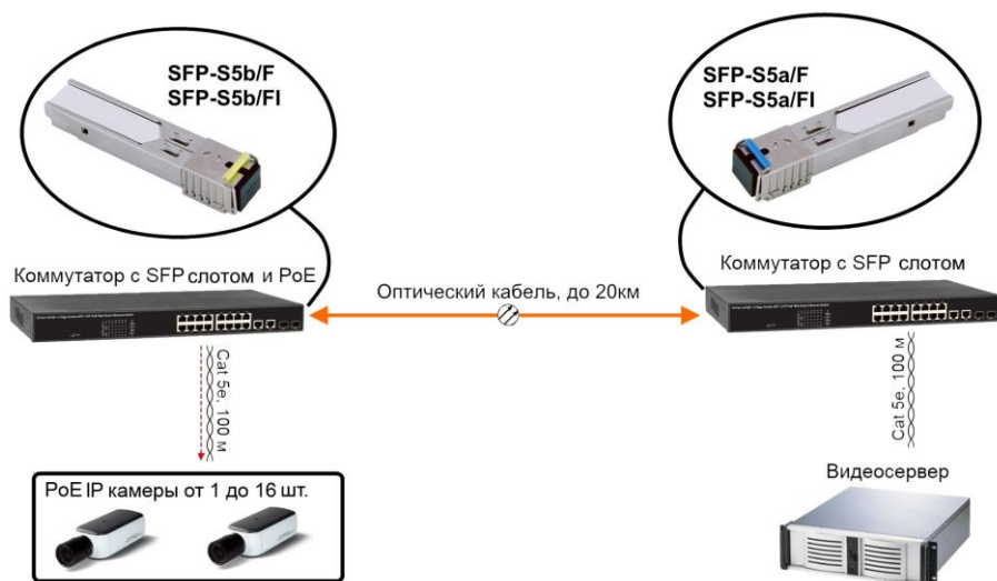
Рис. 4 Схема подключения SFP-модулей
